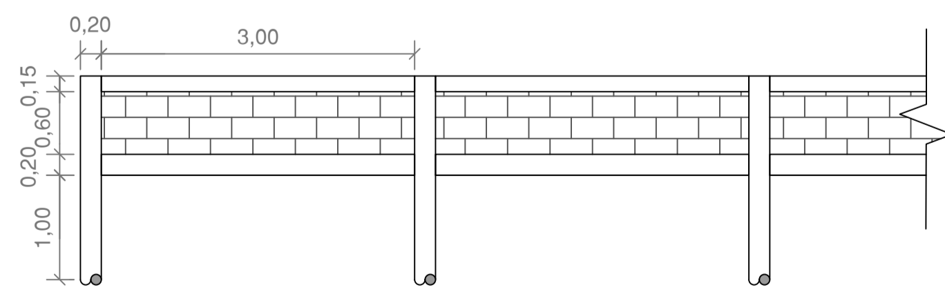
DETALHE ESTACAS, VIGAS, PILARES E ALVENARIA TRECHO P04-P05 ESC.: 1:50
