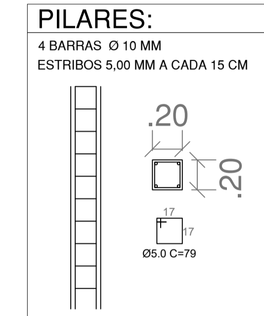
ARMADURA PILARES ESC.: 1:25
