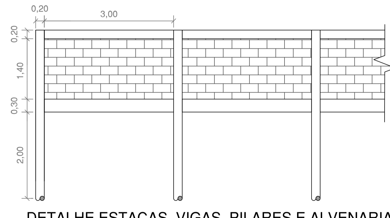
DETALHE ESTACAS, VIGAS, PILARES E ALVENARIA TRECHO P02-P03 ESC.: 1:50
