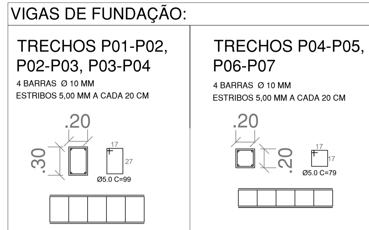
ARMADURA VIGAS DE FUNDAÇÃO ESC.: 1:25
