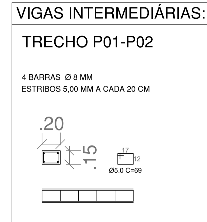
ARMADURA VIGAS INTERMEDIÁRIAS ESC.: 1:25
