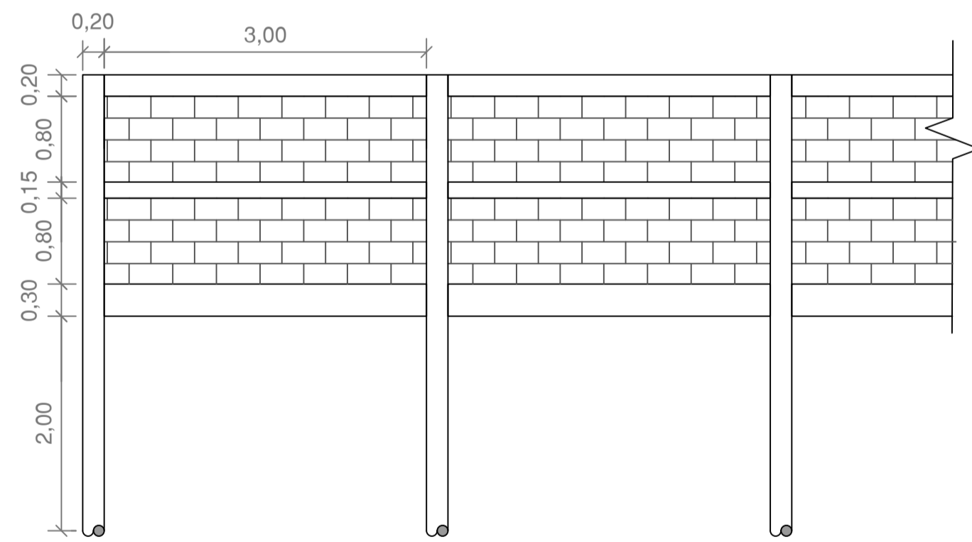
DETALHE ESTACAS, VIGAS, PILARES E ALVENARIA TRECHO P01-P02 ESC.: 1:50
