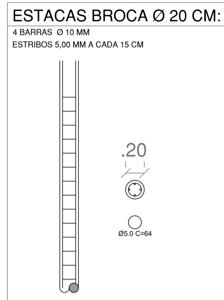
ARMADURA ESTACAS BROCA ESC.: 1:25
