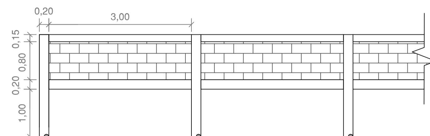
DETALHE ESTACAS, VIGAS, PILARES E ALVENARIA TRECHO P06-P07 ESC.: 1:50
