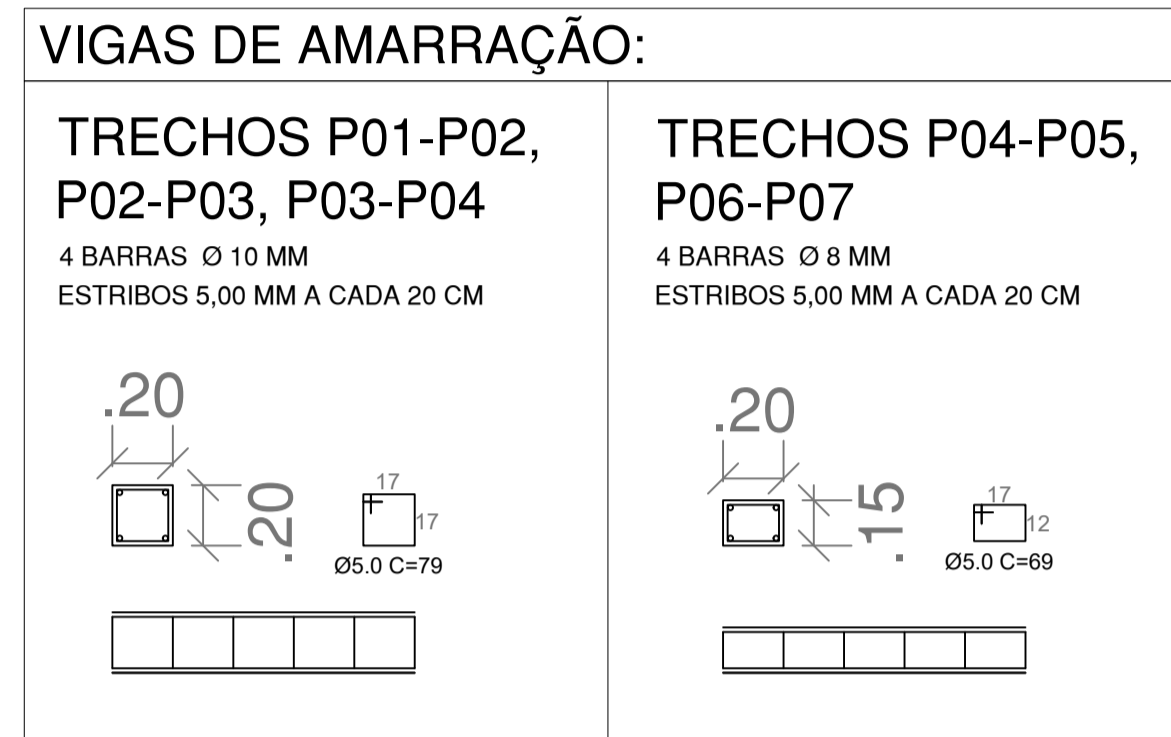
ARMADURA VIGA DE AMARRAÇÃO ESC.: 1:25
